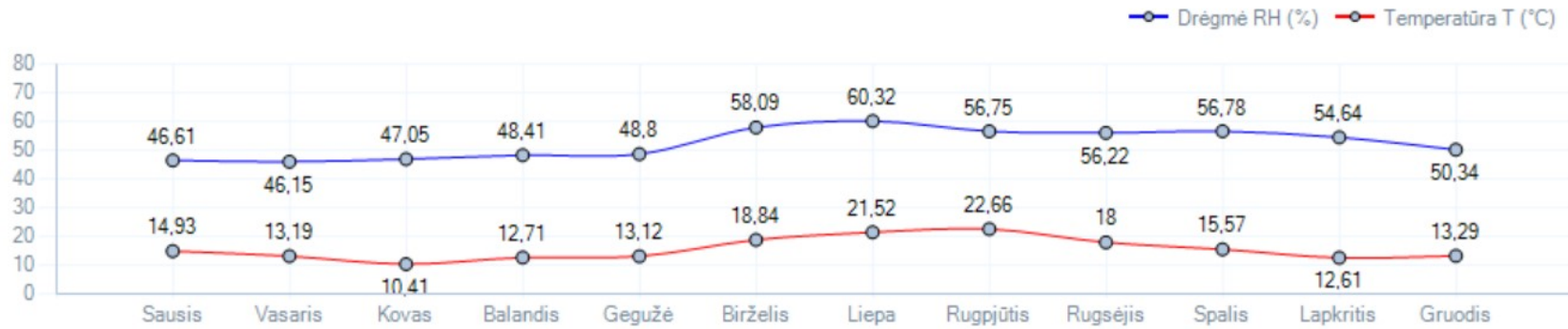
7 saugyklos vidutinē temperatūra ir santykinē drēgmē
